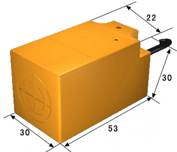
GH1电感式接近开关 ( )
