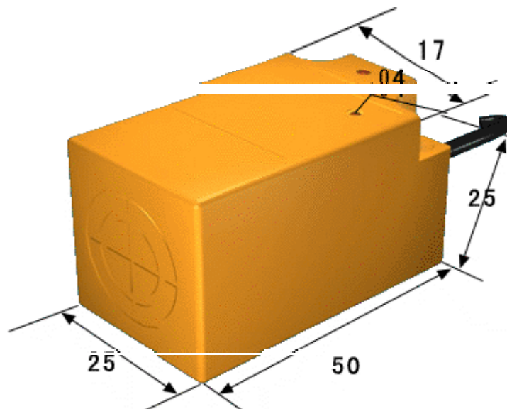
GH1 电感式接近开关 ( )
