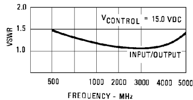
VSWR
