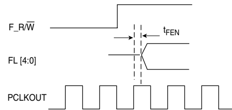
Fig. 12c Flag Port Enable Time
