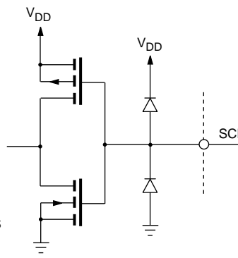
Fig. 3 Pin 14 SCE
