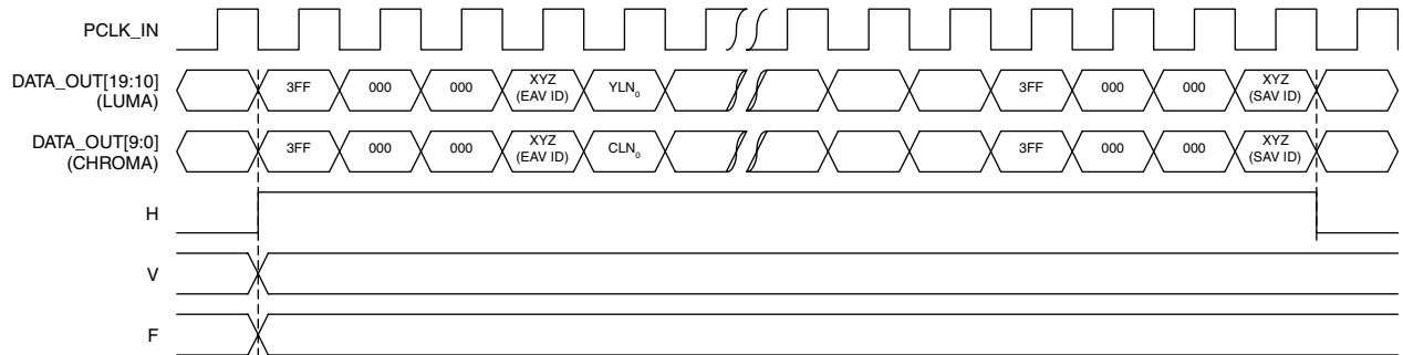
Fig. 2 HVF Timing
