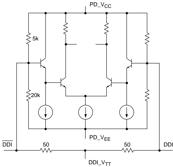
Fig. 1 DDI/DDI Input
