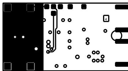
Fig. 28 Bottom Copper Layer
