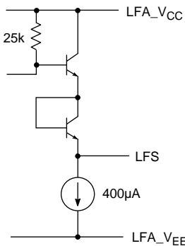
Fig. 6 LFS Output
