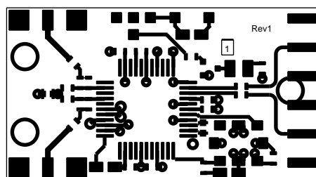
Fig. 26 Top Copper Layer
