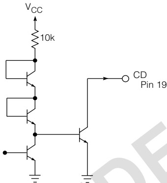
Fig. 7 Pin 19
