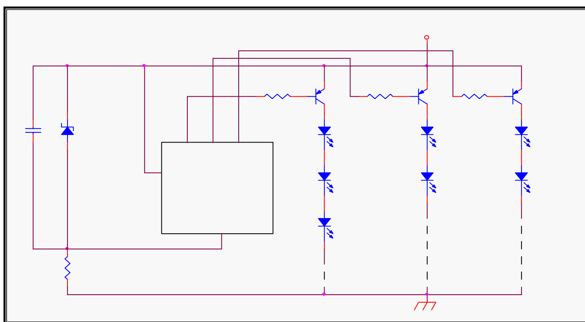
12V 之應用線路一
