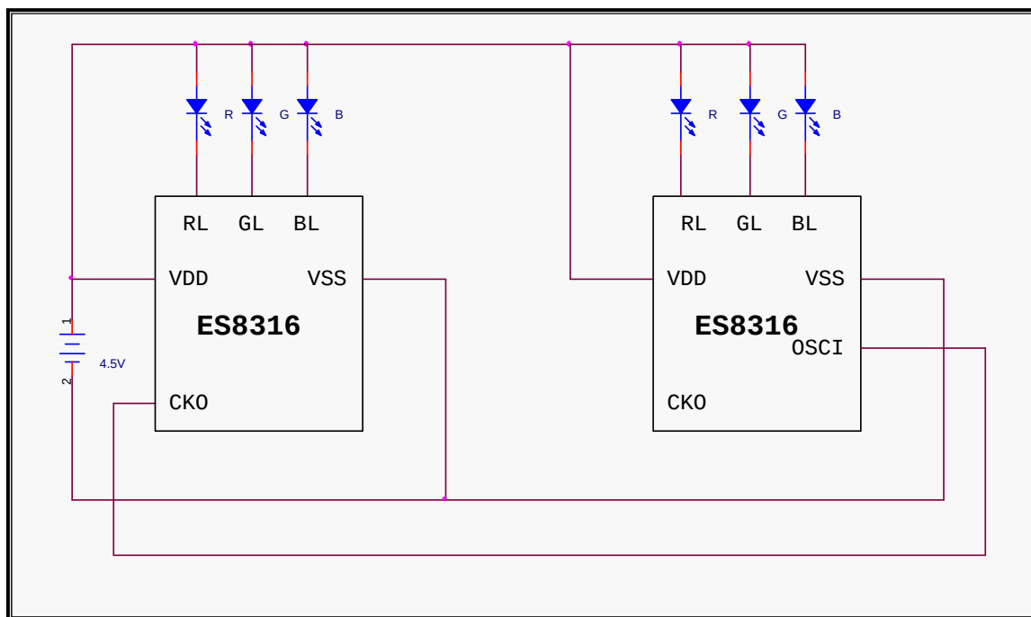
串聯同步應用線路圖
