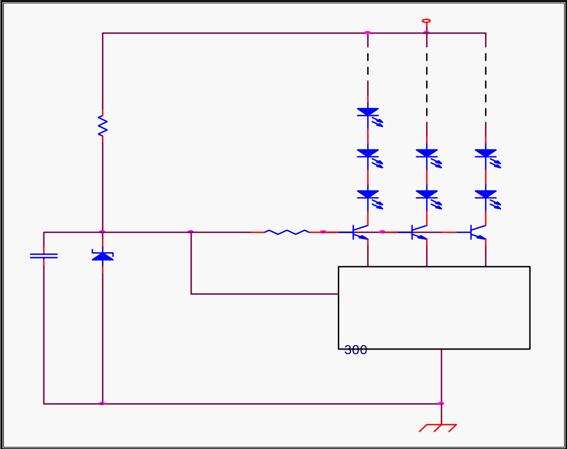
燈串之應用線路一
