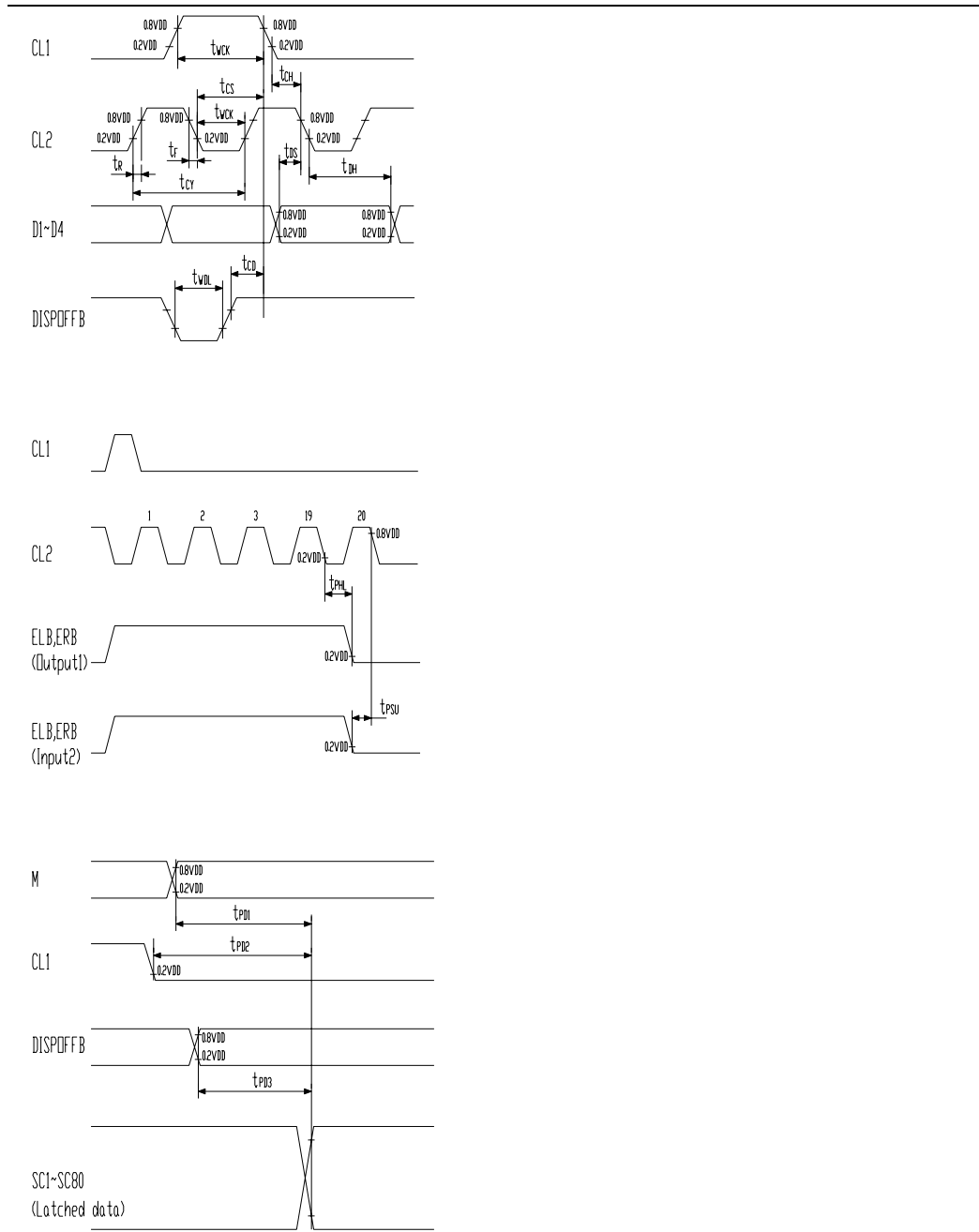
5-2-2. 行驱动时序及时序图 (VCC=5.0V ± 10%, VSS=0V, Ta=-30 to +85 °C)
