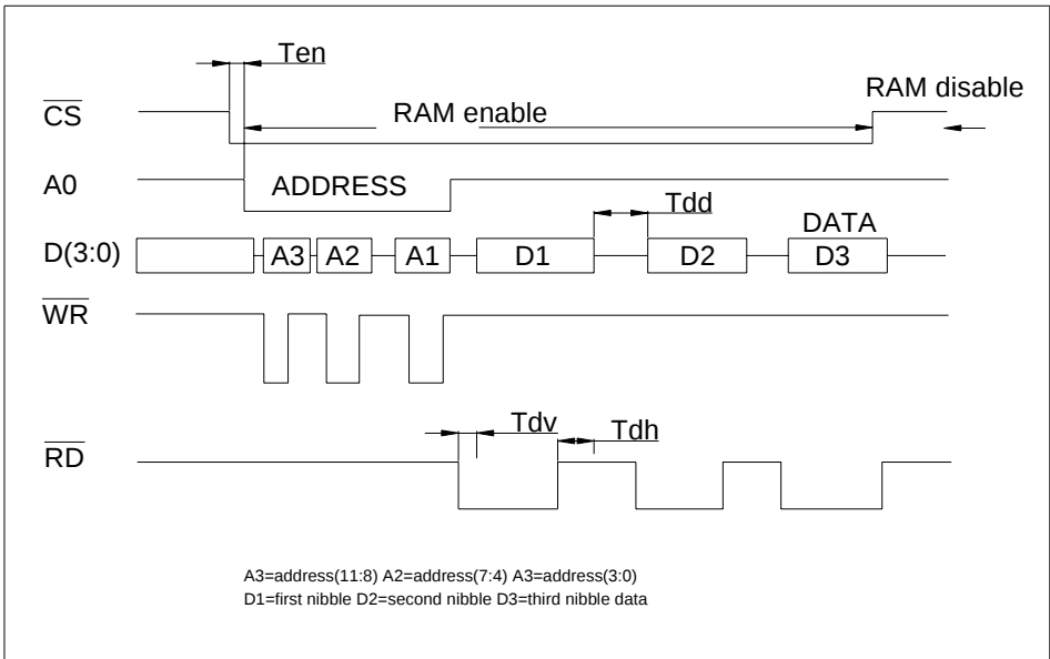
(b) 读时序图
