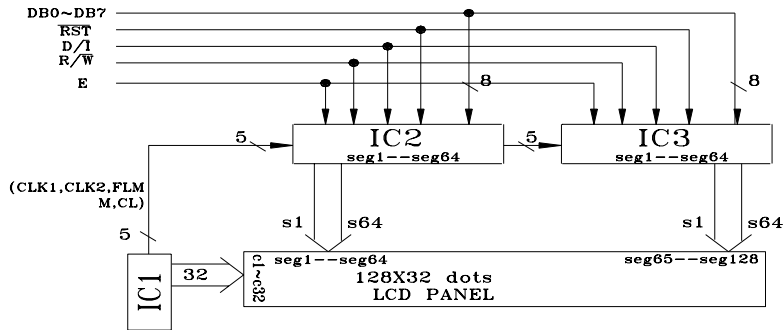
Fig. 5-4 逻辑图
