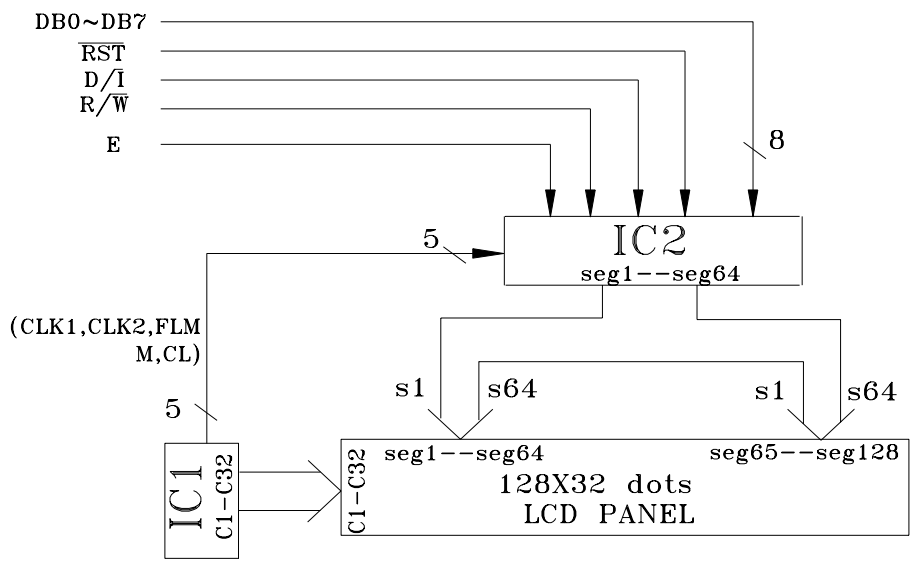
Fig.5-4逻辑图
