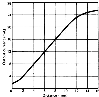
M30 Size Sensor E2CA-X10A
