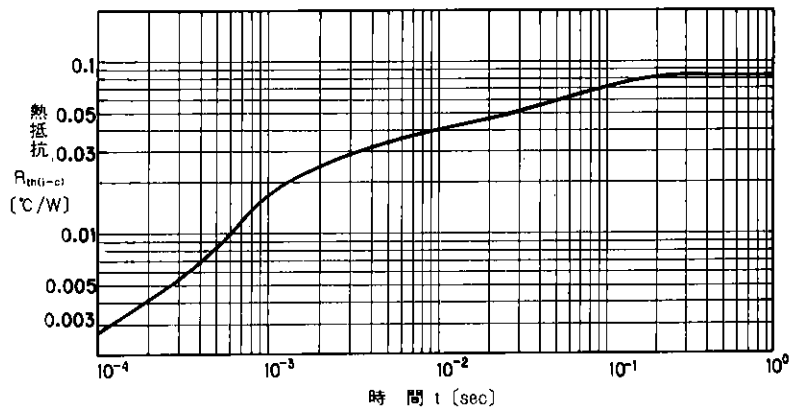
過渡熱抵抗(トランジスタ)特性
