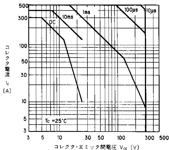
安全動作領域特性
