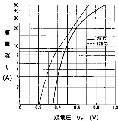
順特性
