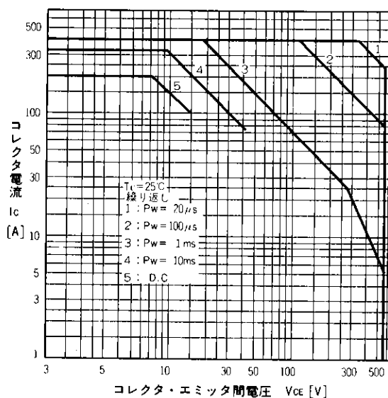
安全動作領域特性(繰り返し) Safe Operating Area
