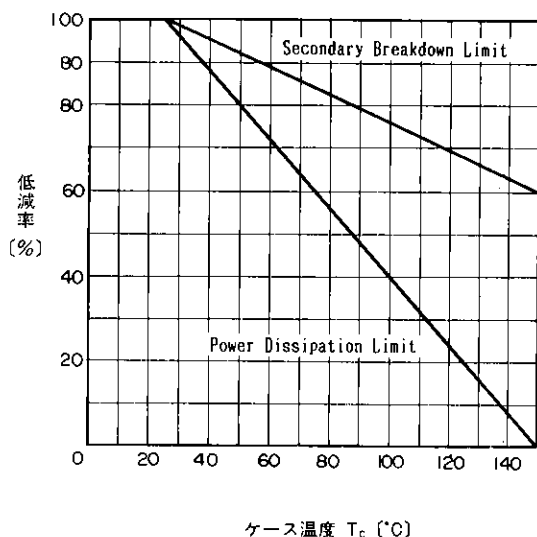
ASO 低減特性 ASO Derating
