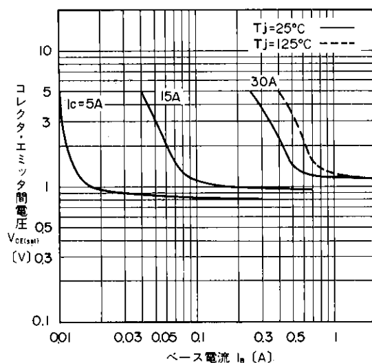
出力特性
