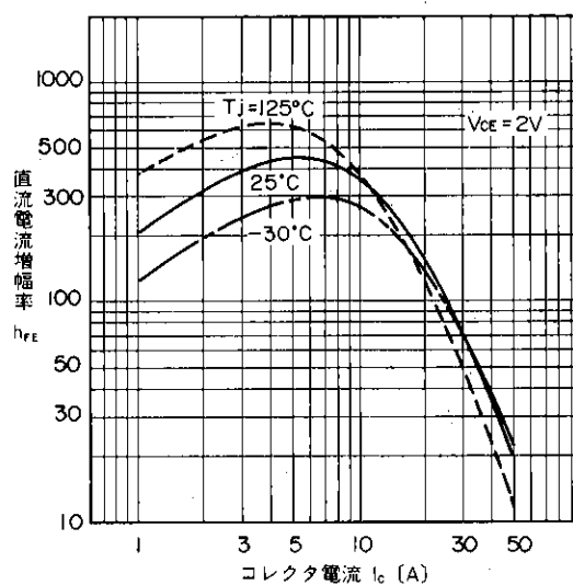
直流電流増幅率—コレクタ電流特性
