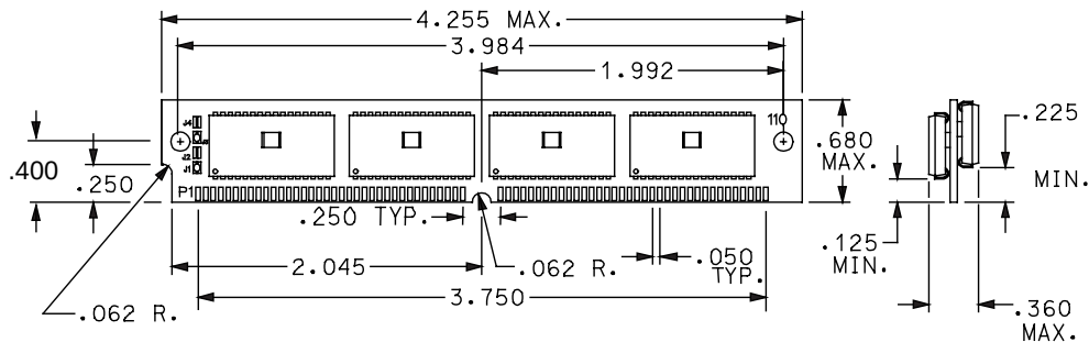
176-8F321024C Pkg.
