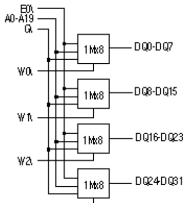
EDI7F33IMC-BNC 1Megx32 80 pin SIMM
