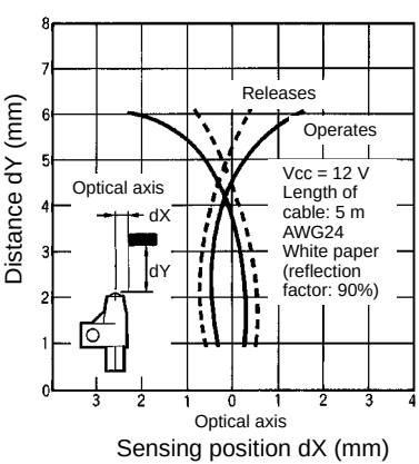
EE-SPZ301Y-01, EE-SPZ401Y-01
