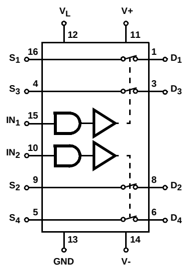
DG405
