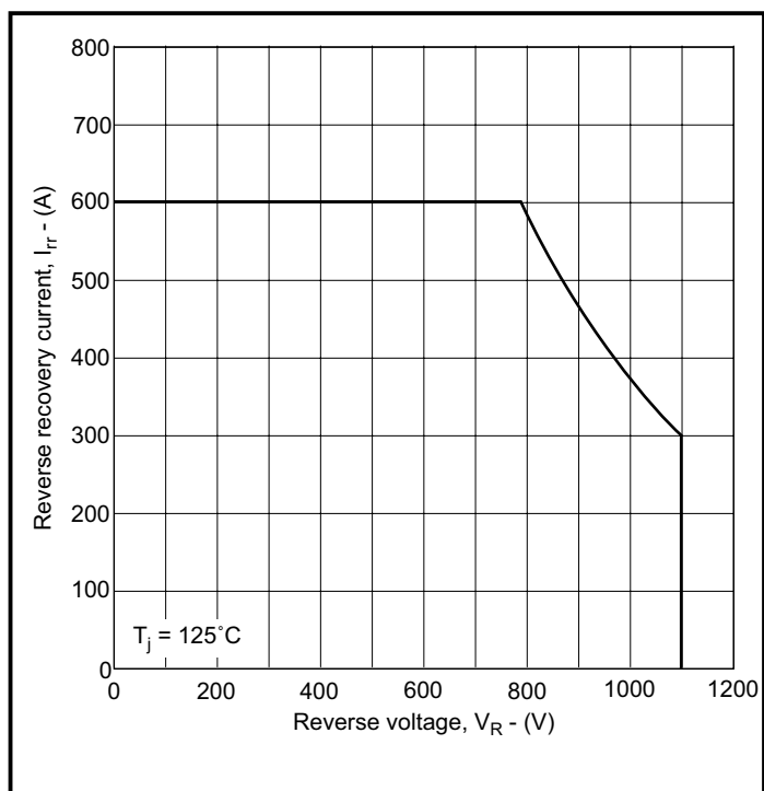
Fig. 7 RBSOA
