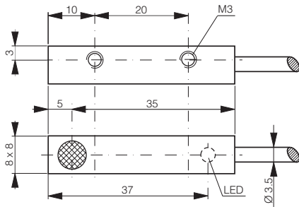
DW-AD-50#-C8
