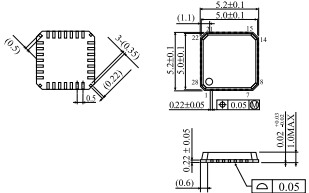
VQFN28
