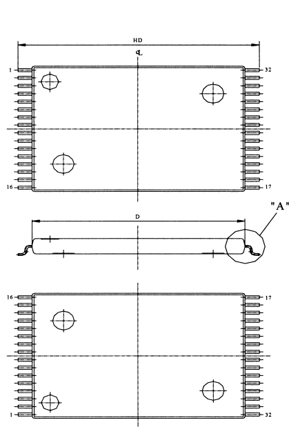
STSOP - 32
