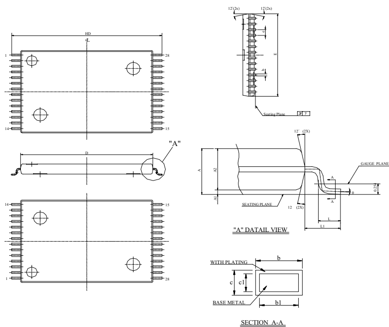
TSOP - 28
