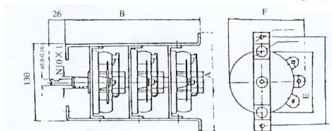
BC1D-150/3 瓷盘式变阻器外形及安装尺寸
