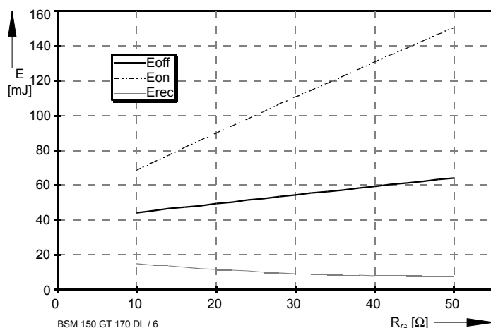
Bild / Fig. 6 Schaltverluste (typisch) / Switching losses (typical) E_{on} = f(R_G) , E_{off} = f(R_G) , E_{rec} = f(R_G) I_C = 150A , V_{CE} = 900V , T_J = 125^\circ C
