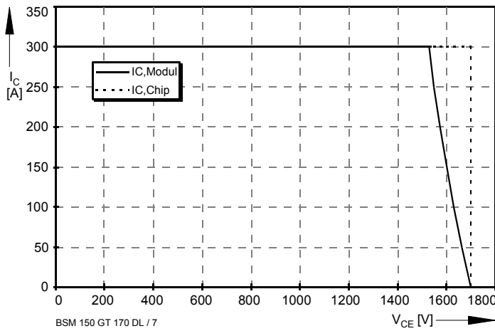
Bild / Fig. 7 Sicherer Arbeitsbereich (RBSOA) / Reverse bias safe operation area (RBSOA) R_g = 10\Omega , T_{vj} = 125^\circ\text{C}
