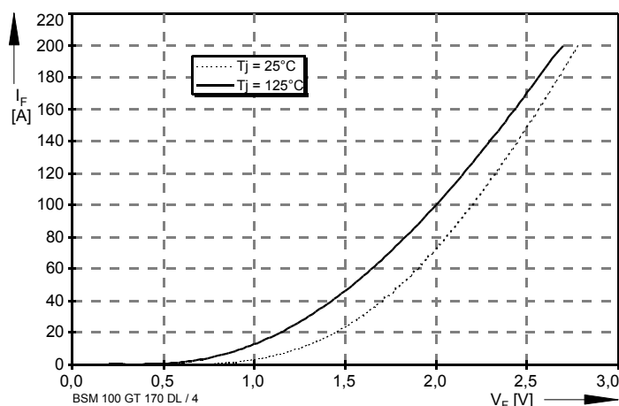
Bild / Fig. 4 Durchlaßkennlinie der Inversdiode (typisch) / Forward characteristic of inverse diode (typical) I_F = f(V_F)
