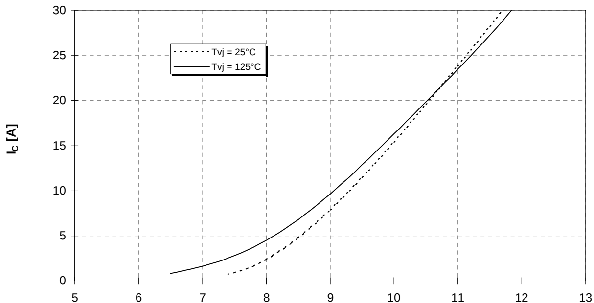
Übertragungscharakteristik (typisch) Transfer characteristic (typical)
