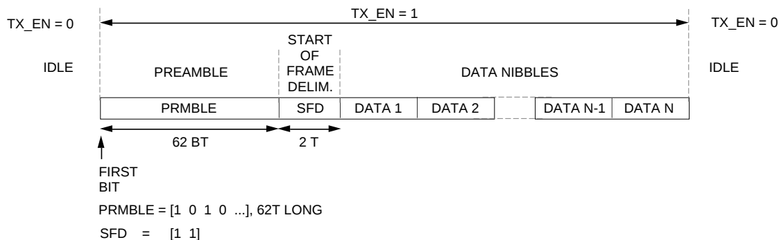
a.) MII Frame Format
