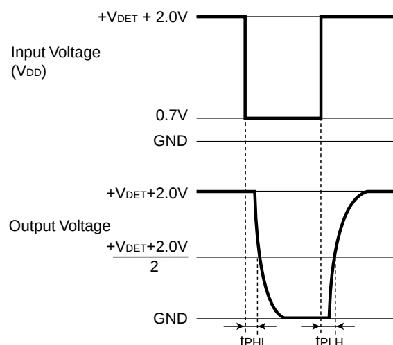
CMOS Output
