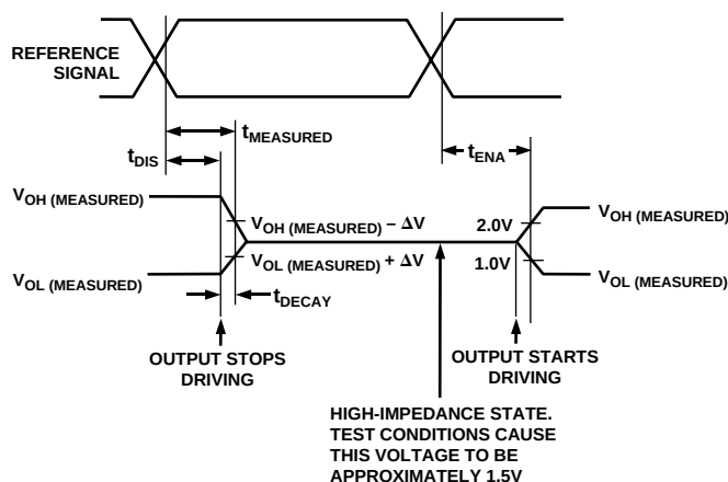
Figure 28. Output Enable/Disable
