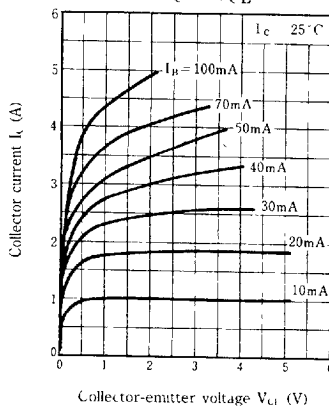
I_C - V_{CE}
