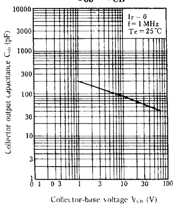
C_{ob} - V_{CB}
