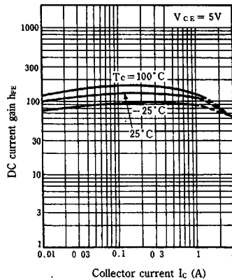
h_{FE} - I_C
