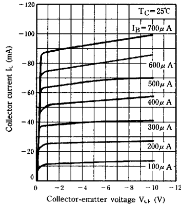
I_C - V_{CE}
