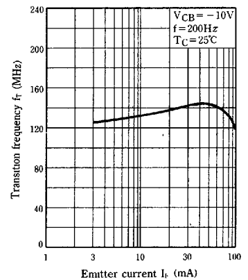
f_T - I_E
