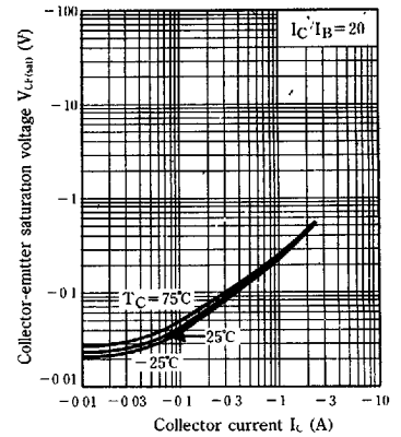
V_{CE(sat)} - I_C
