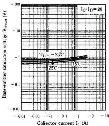
V_{BE(sat)} - I_C
