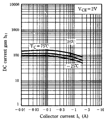
h_{FE} - I_C
