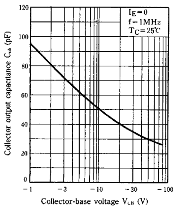
C_{ob} - V_{CE}
