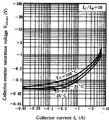
V_{CE(sat)} - I_C
