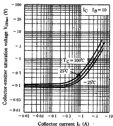
V_{CE(sat)} - I_C
