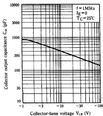
C_{ob} - V_{CB}
