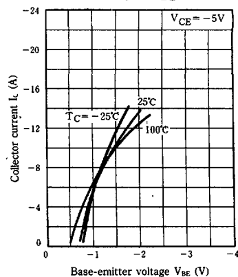
I_C - V_{BE}
