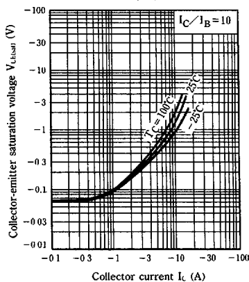
V_{CE(sat)} - I_C
