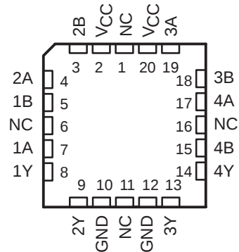
54ACT11002 . . . FK PACKAGE
