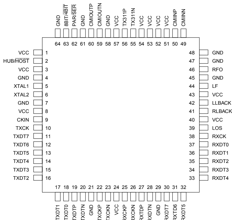
64-Pin TQFP (JEDEC LQFP) 78P2254-IGT
