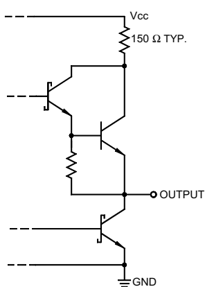
TTL OUTPUT CIRCUIT
