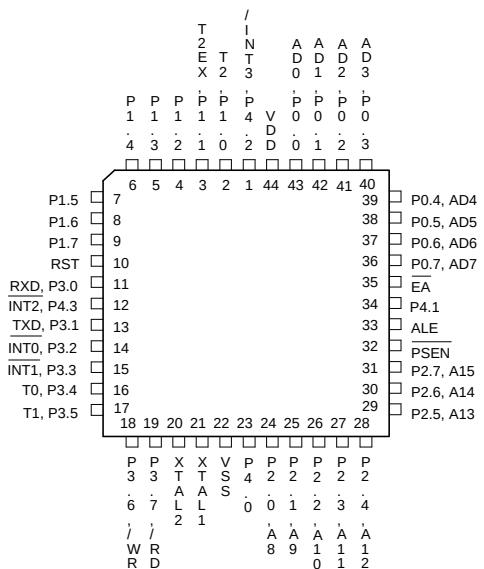
44-Pin PLCC (W78L54P)
