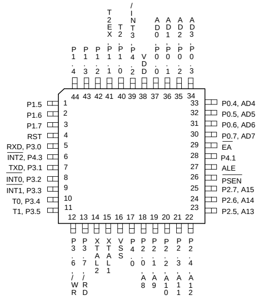
44-Pin QFP (W78L54F)
