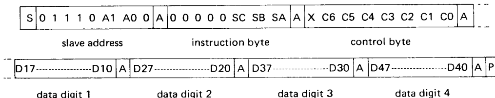
Fig. 3b I 2 C-Bus format; WRITE mode.
