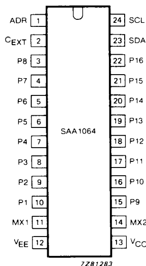
Fig.2 Pinning diagram.
