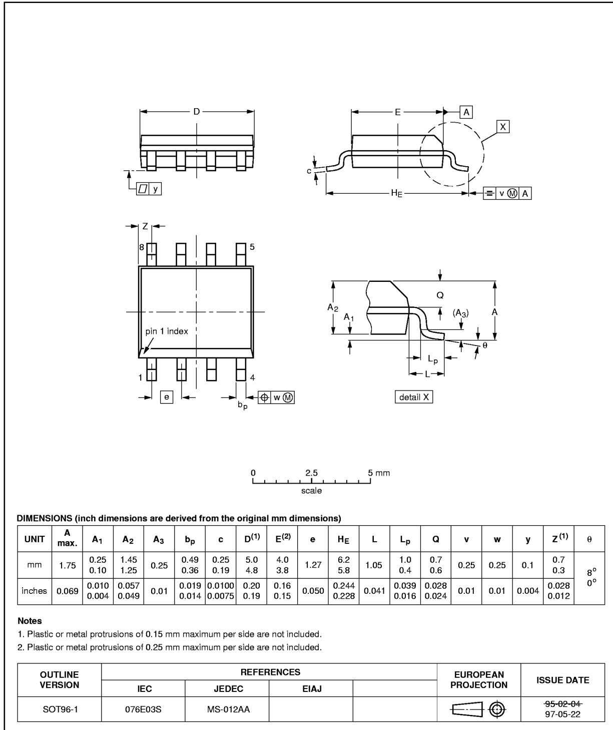
Fig 20. SOT96-1.
