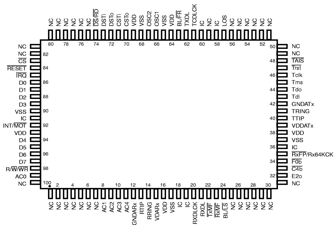
100 PIN MQFP (JEDEC MO-112)
