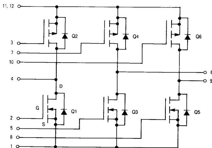
MPM3003 Schematic
