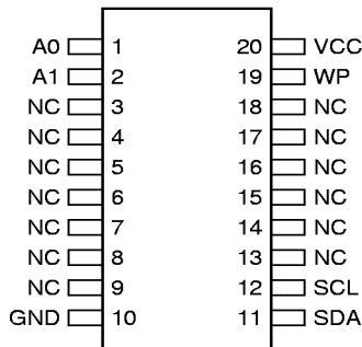
20-Pin SOIC
